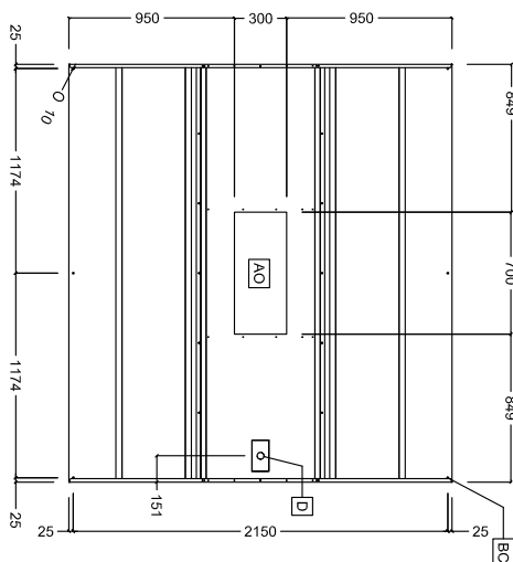
Boven aanzicht
